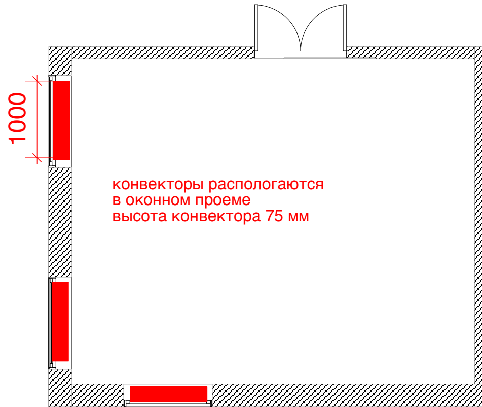
План расположения конвекторов
